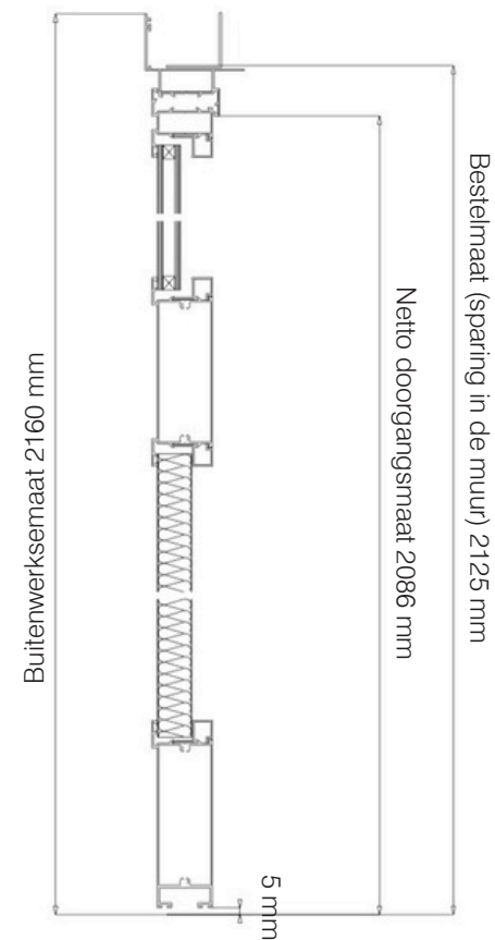
Zij-aanzicht (AA)
