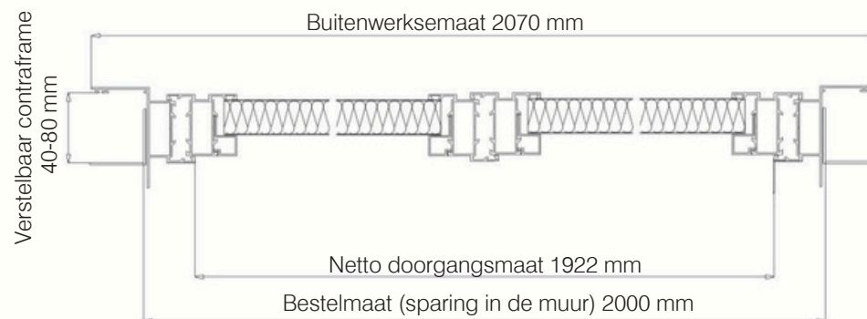
Bovenaanzicht (BB)
