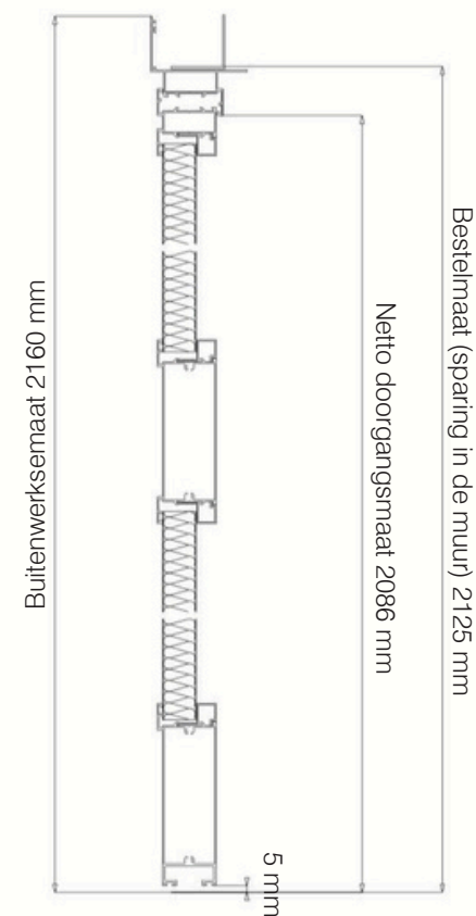
zij-aanzicht (AA)
