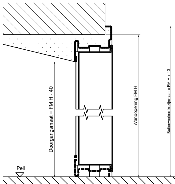
Verticale doorsnede
